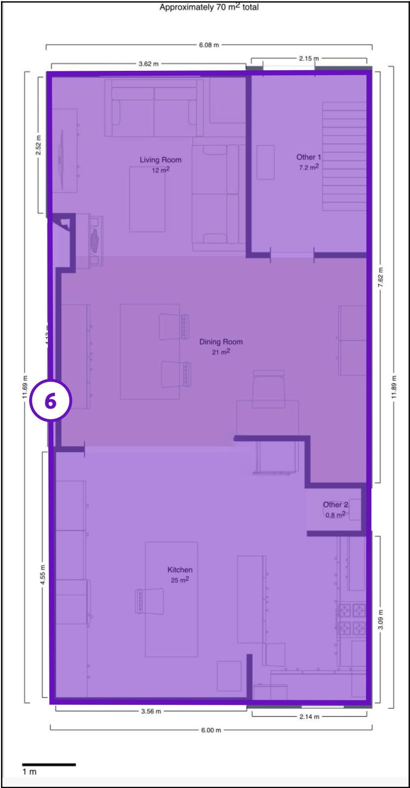
Legende van plan 1.6: Gelijkvloers kopie kopie
