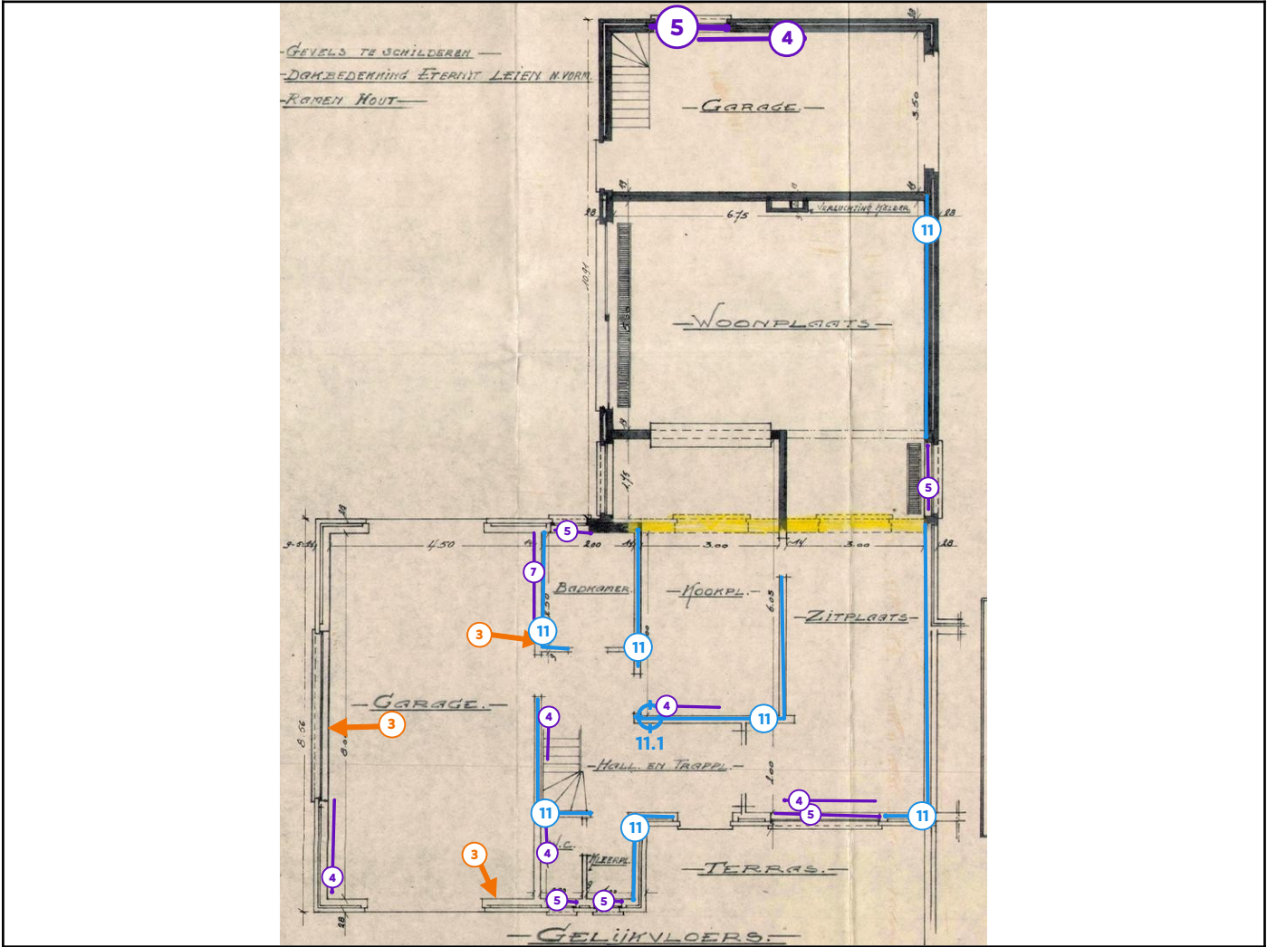
Legende van plan 1.1: Gelijkvloers hoofdwoonst
