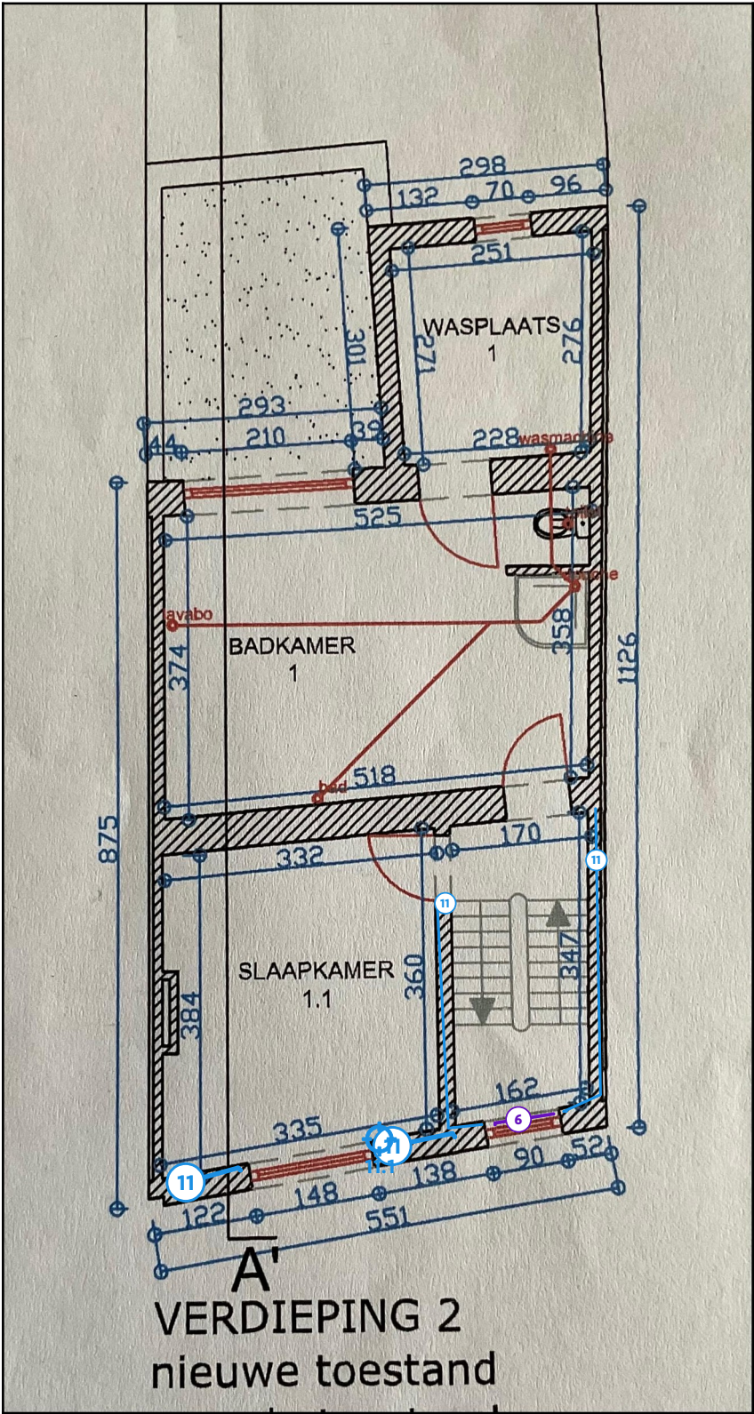
Legende van plan 1.7: 2de verdiep
