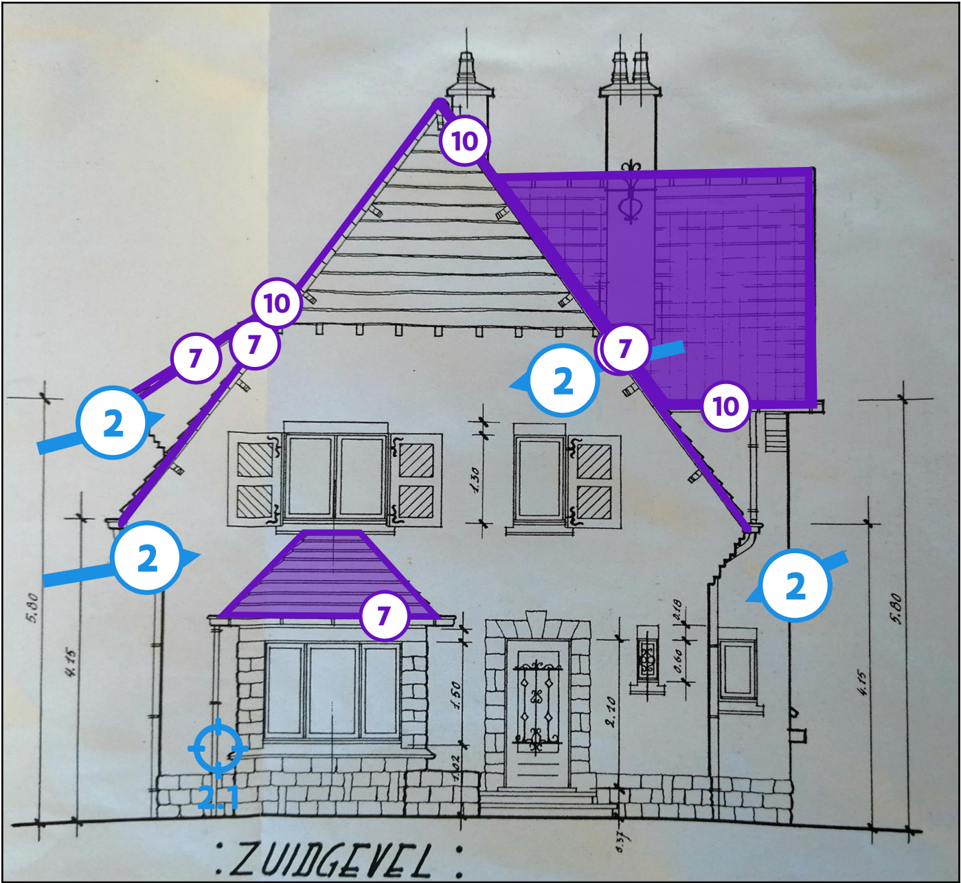
Legende van plan 1.7: gevel voor
